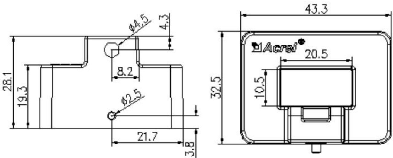
图 5 ADW350WD 配套霍尔电流传感器 AHKC-BS 尺寸图
