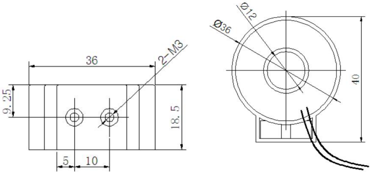
图 4 ADW350WA 10(50)A 配套互感器尺寸图
