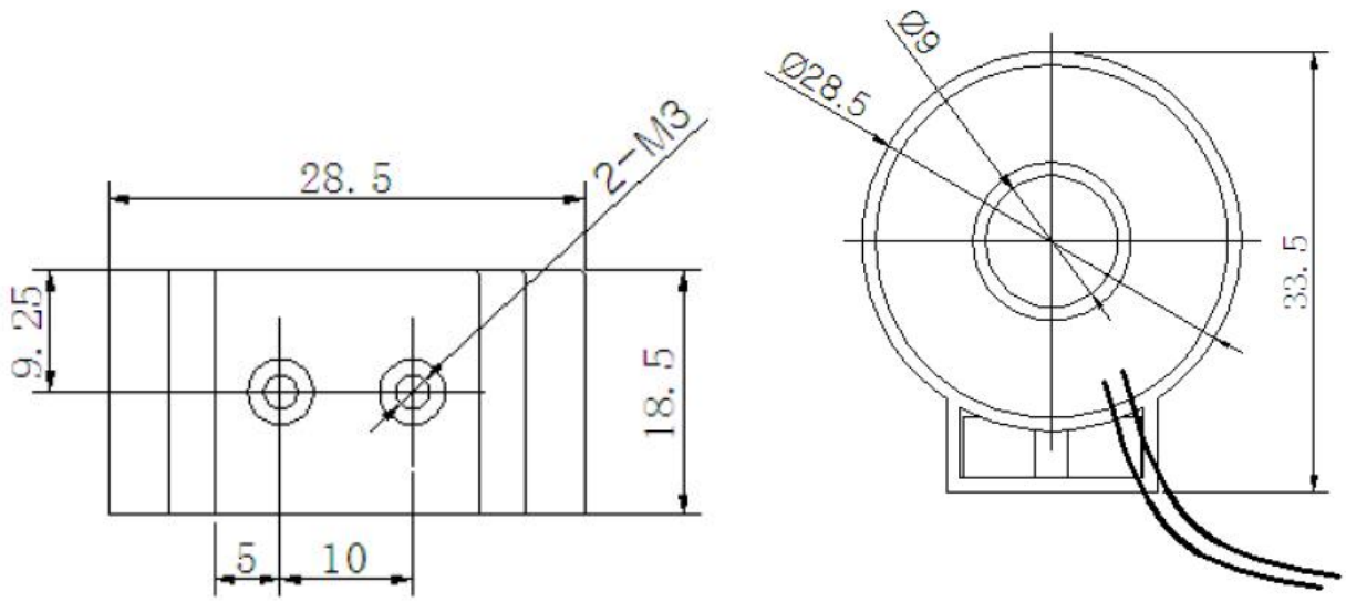
图 3 ADW350WA 20(100)A 配套互感器尺寸图
